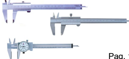
Calibres Mecanicos
